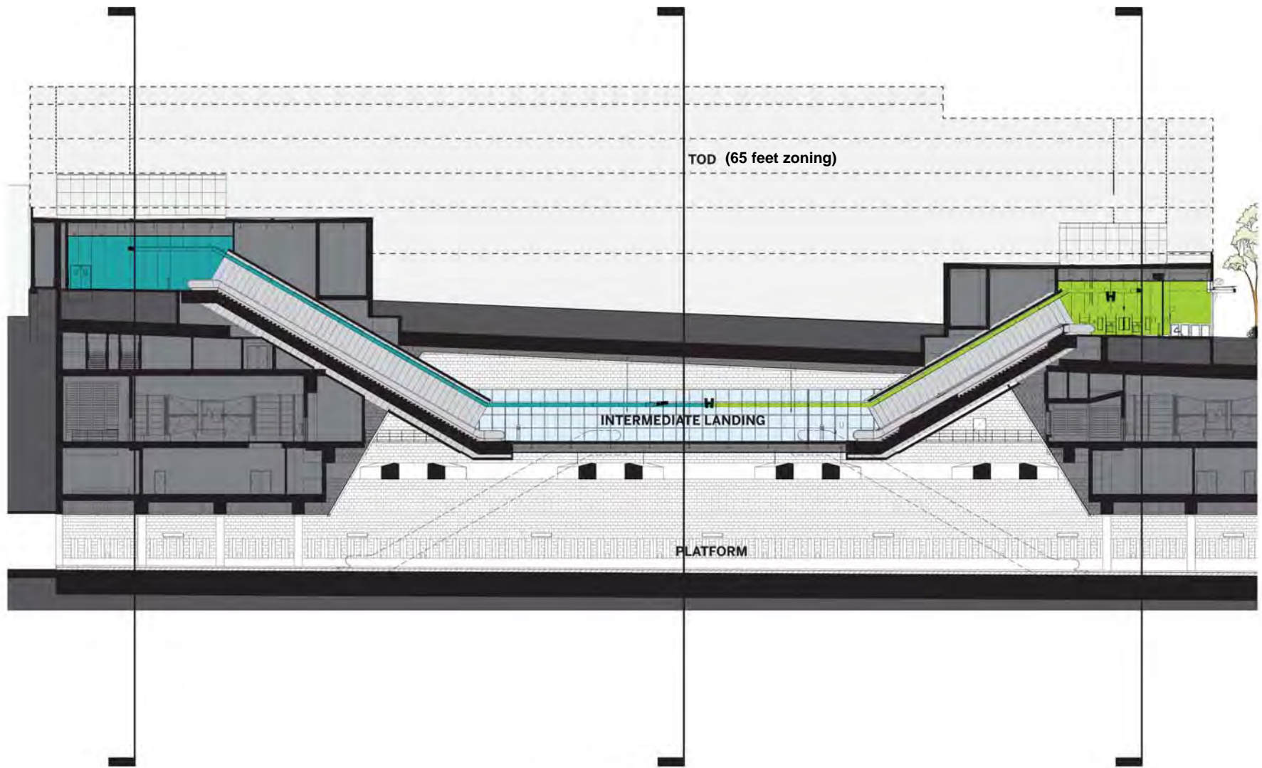
Longitudinal Section
