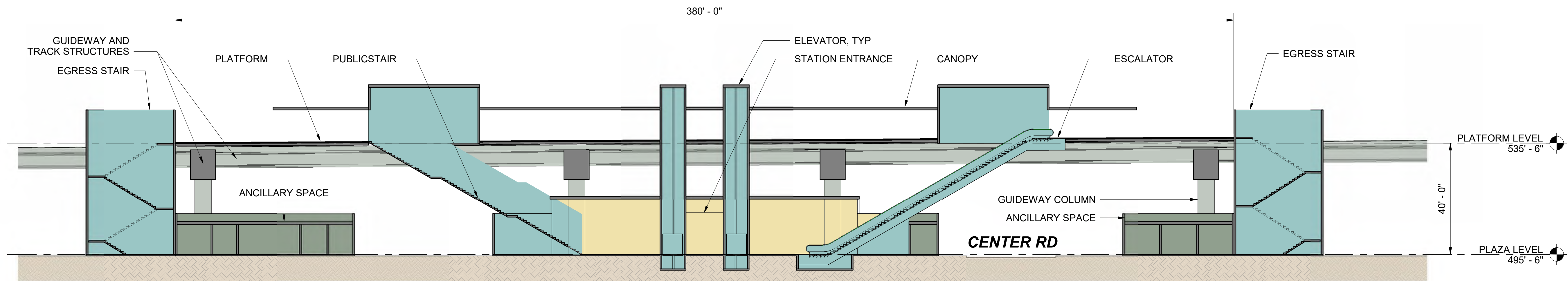
AIR-A LONG SECTION
