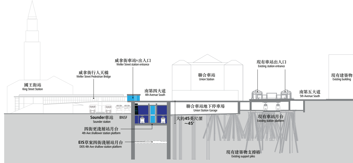
橫切圖 D Section D
