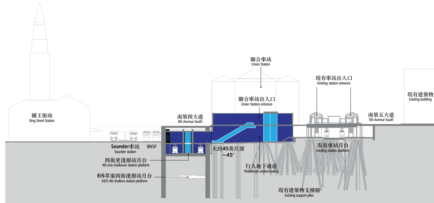
橫切圖 C Section C
