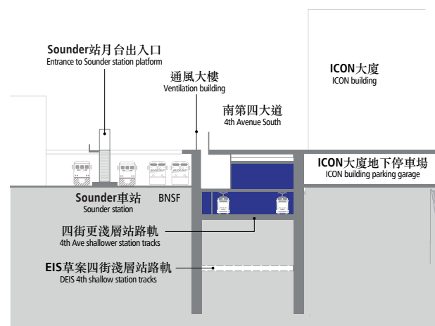
橫切圖 B Section B
