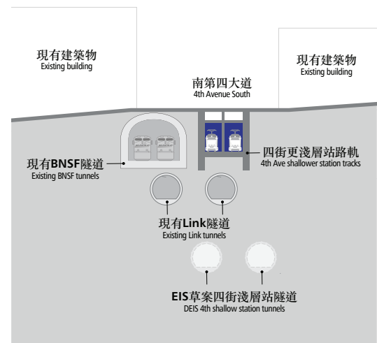
橫切圖 A Section A
