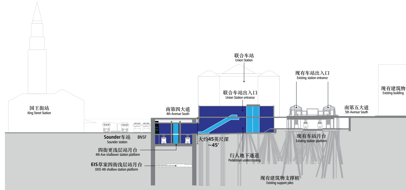
横切图 C Section C
