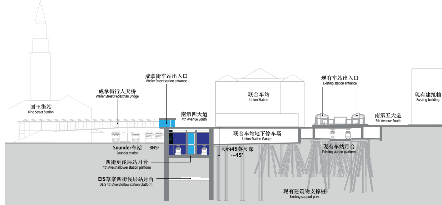
横切图 D Section D
