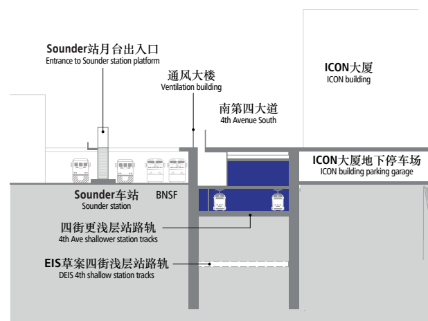
横切图 B Section B
