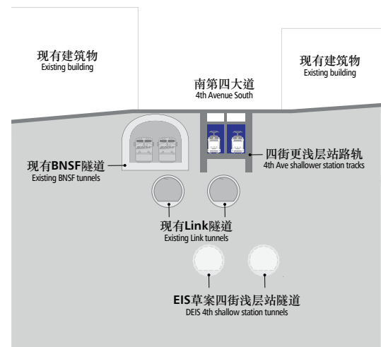
横切图 A Section A
