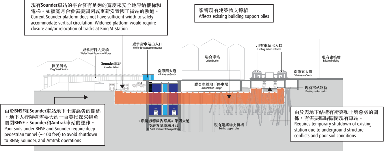
橫切圖 Section
