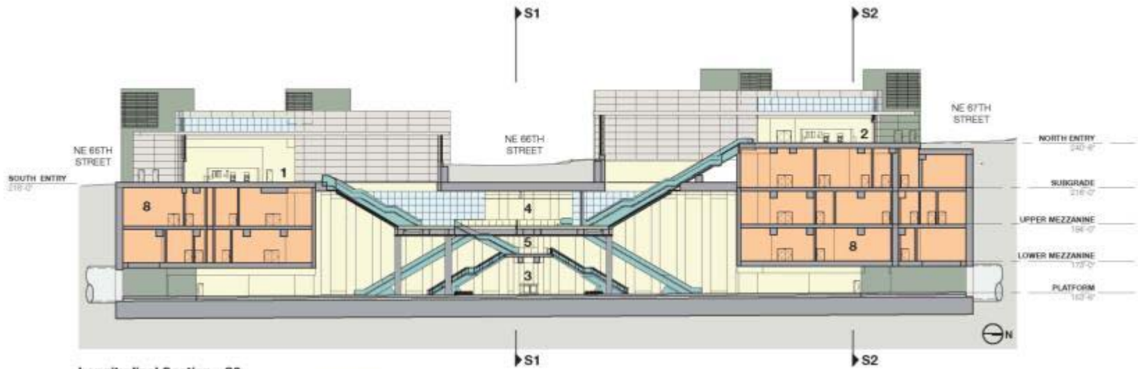
Longitudinal Section - S3
